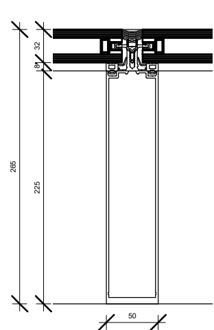
3 Detail 2 1 : 5
