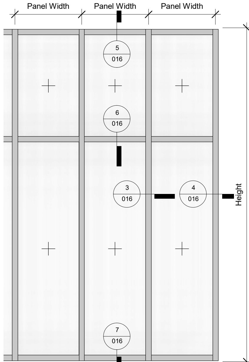
2 Elevation Back 1 : 20
