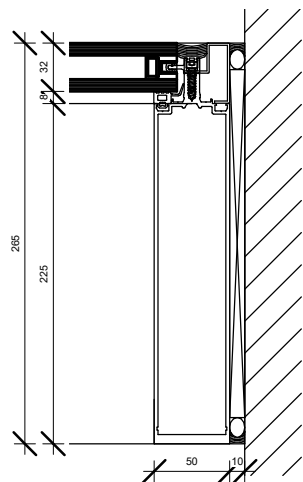
4 Detail 1 1 : 5
