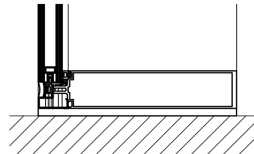
7 Detail 5 1 : 5
