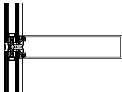
6 Detail 4 1 : 5
