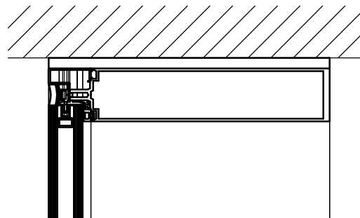
5 Detail 3 1 : 5
